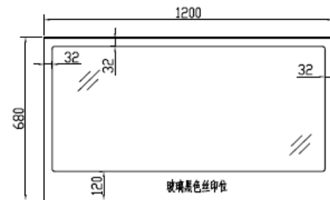
PLAN 顶视图
