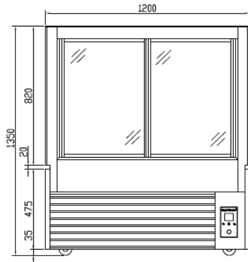
BACK 后视图
