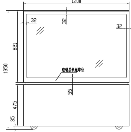
ELEVATION 前视图
