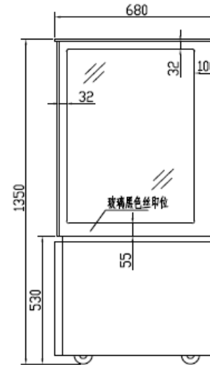
SIDE VIEW 左视图
