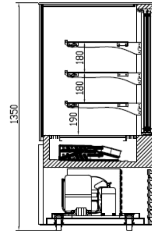
SECTION VIEW 左侧剖视图
